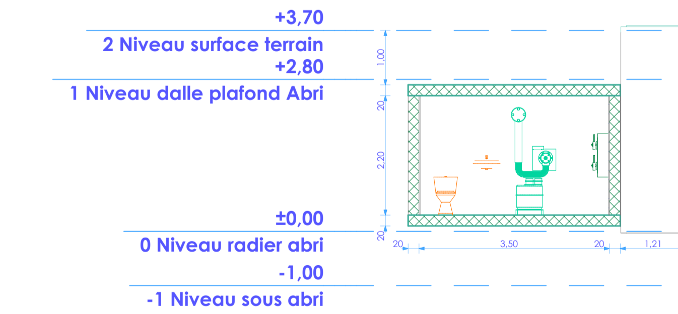
B3 Coupe BB 1:70,00
