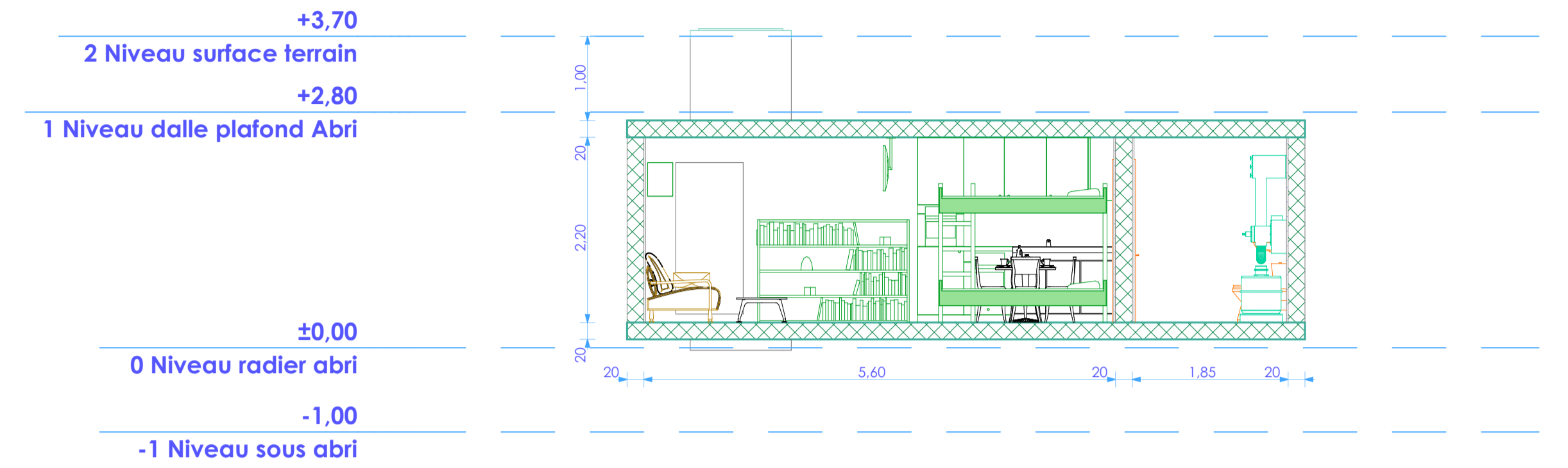
B1 Coupe BB 1:57,59
