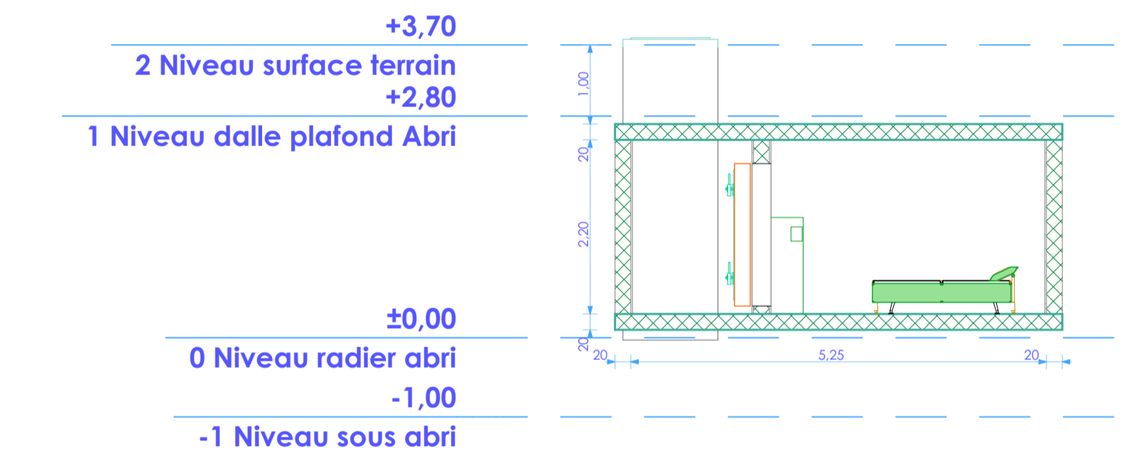
B2 Coupe BB 1:67,84
